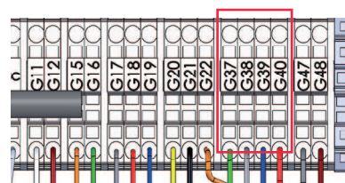
Connettere a G37-G40 sulla morsettieria del sensore. Utilizzare almeno un cavo da 0,5 mm 2 .
